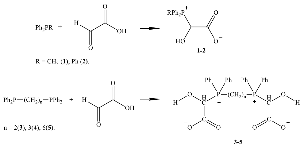
Схема 1. Синтез карбоксилатных фосфабетаинов на основе глиоксиловой кислоты
